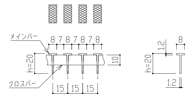
TBノンスリップ(ローレット) h=20 p=15 【メインバー詳細図】
