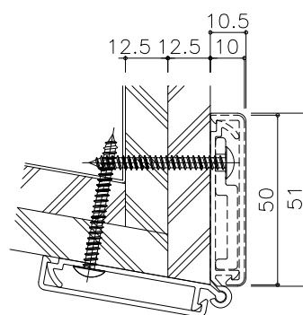
70° コーナー納まり例
