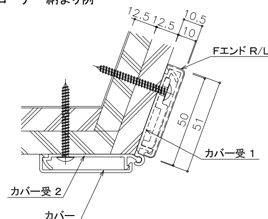
110° コーナー納まり例
