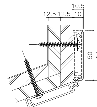
110° コーナー納まり例
