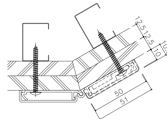
150° コーナー納まり例
