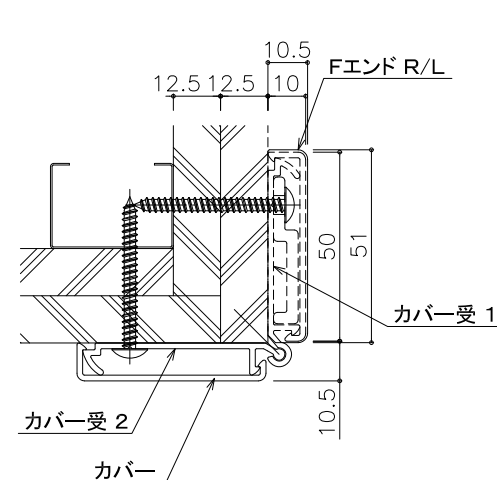
90° コーナー納まり例
