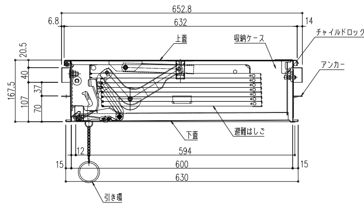
A-A矢視図
