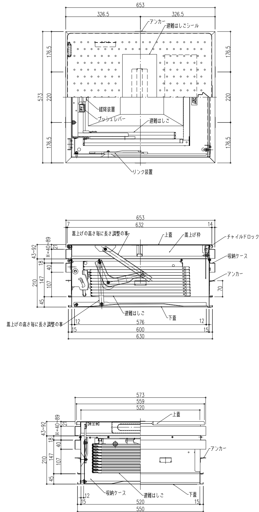
収納状態 S=1/10
