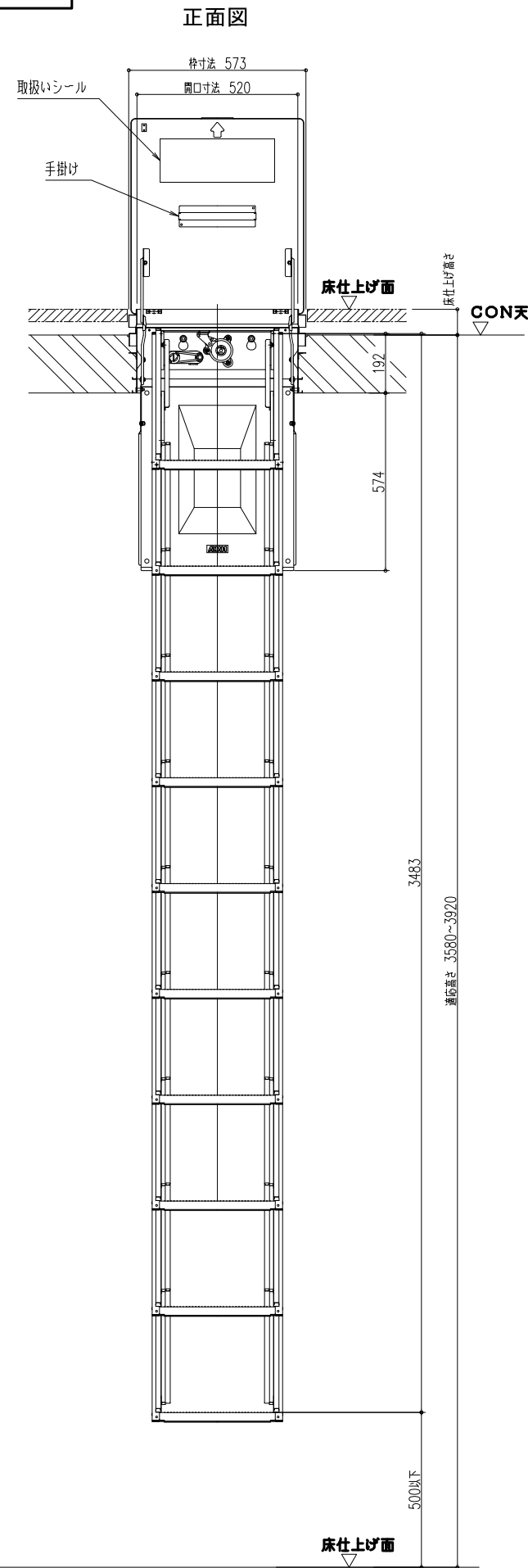
展張状態 S=1/20
