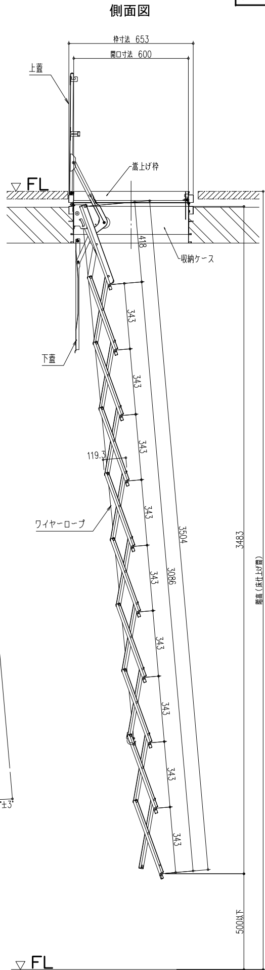
展張状態 S=1/20
