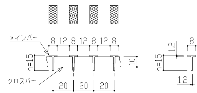
TBノンスリップ(ローレット) h=15 p=20 【メインバー詳細図】
