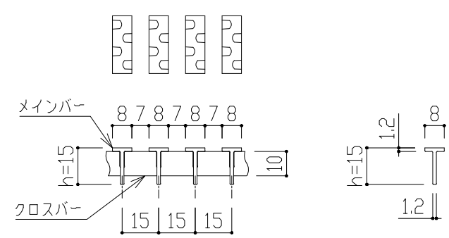
TBノンスリップ(エンボス) h=15 p=15 【メインバー詳細図】
