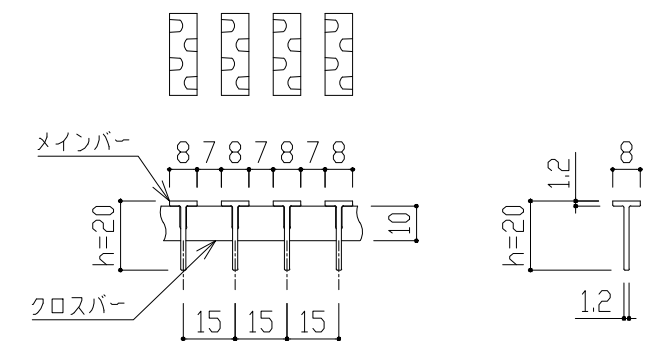
TBノンスリップ(エンボス) h=20 p=15
