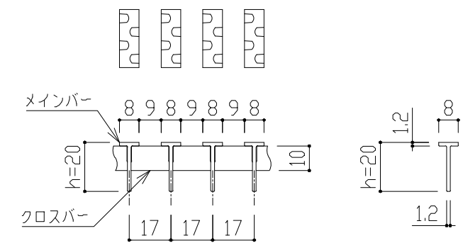
TBノンスリップ(エンボス) h=20 p=17 【メインバー詳細図】
