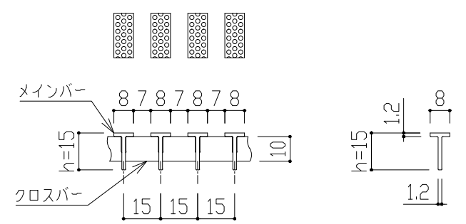
TBノンスリップタイプ(コラムドット) h=15 p=15 【メインバー詳細図】
