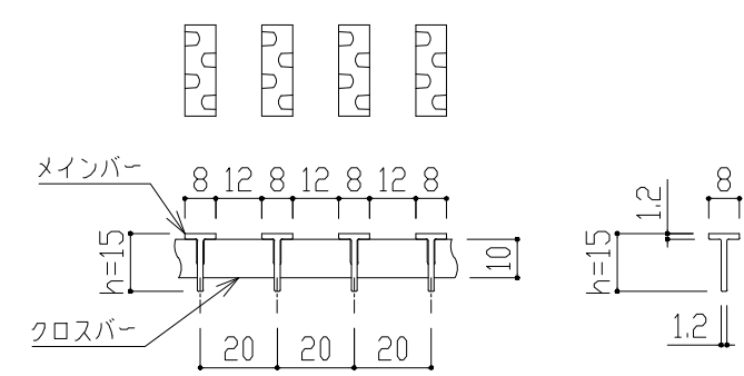
TBノンスリップ(エンボス) h=15 p=20 【メインバー詳細図】
