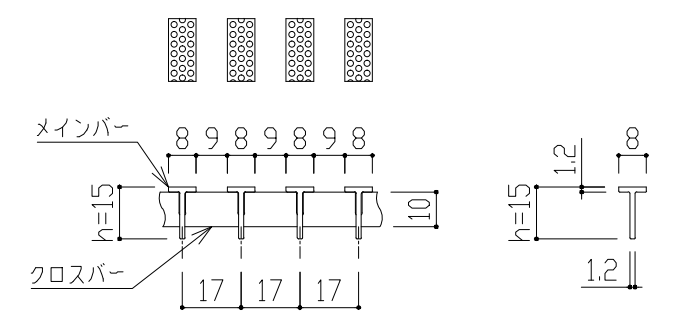
TBノンスリップ(コラムドット) h=15 p=17 【メインバー詳細図】
