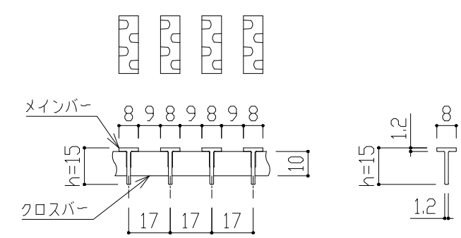
TBノンスリップ(エンボス) h=15 p=17 【メインバー詳細図】
