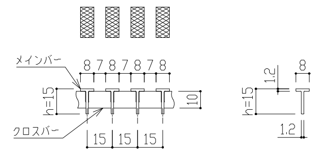
TBノンスリップ(ローレット) h=15 p=15 【メインバー詳細図】
