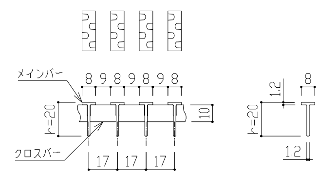
TBノンスリップ(エンボス) h=20 p=17 【メインバー詳細図】
