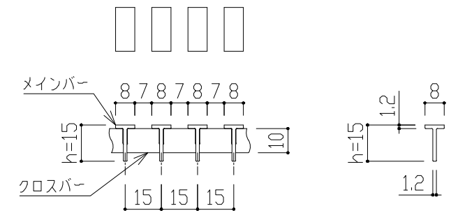
TBプレートタイプ h=15 p=15 【メインバー詳細図】
