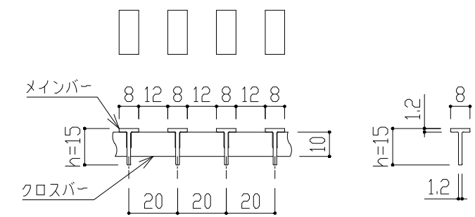
TBプレーンタイプ h=15 p=20 【メインバー詳細図】
