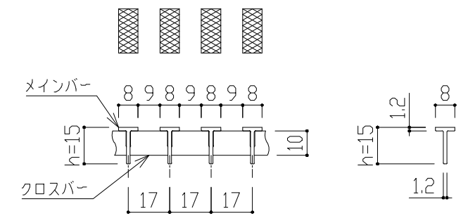
TBノンスリップ(ローレット) h=15 p=17 【メインバー詳細図】
