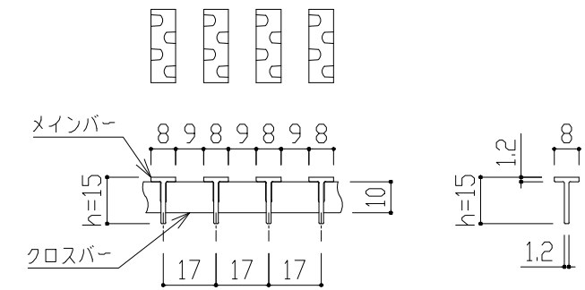
TBノンスリップ(エンボス) h=15 p=17 【メインバー詳細図】
