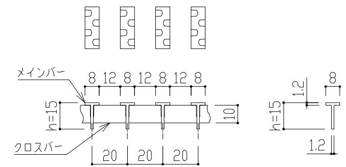
TBノンスリップ(エンボス) h=15 p=20 【メインバー詳細図】
