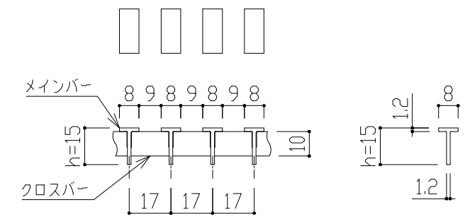
TBプレーンタイプ h=15 p=17 【メインバー詳細図】
