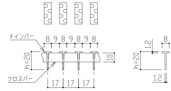
【メインバー詳細図】
