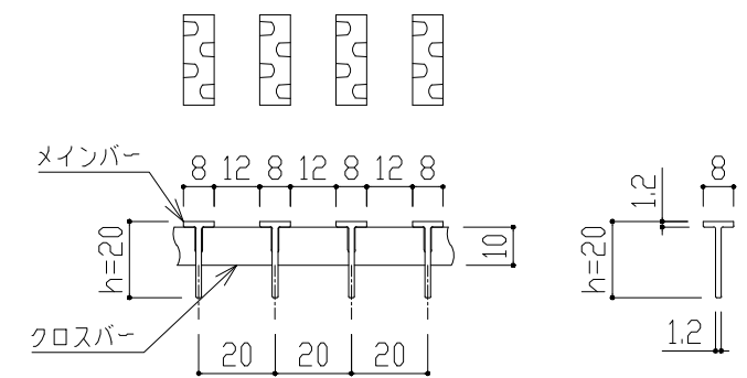
TBノンスリップ(エンボス) h=20 p=20
