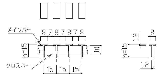
TBプレーンタイプ h=15 p=15 【メインバー詳細図】
