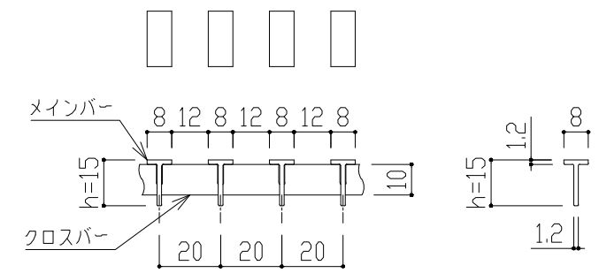
TBプレートタイプ h=15 p=20 【メインバー詳細図】
