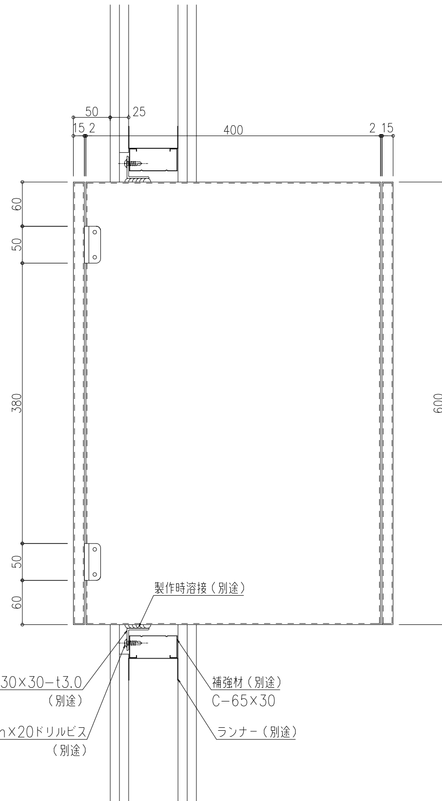
側面図
