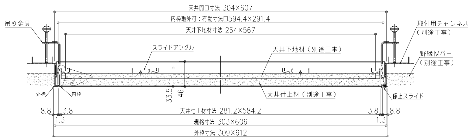
内蓋施工図 S=1/2
