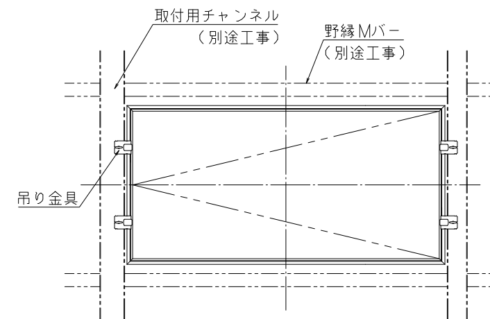
取付状態図 S=1/10
