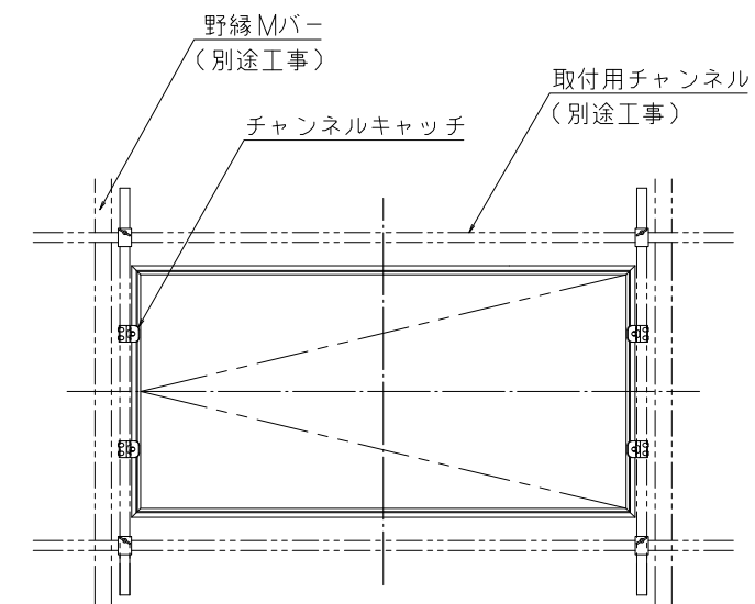
取付状態図 S=1/10
