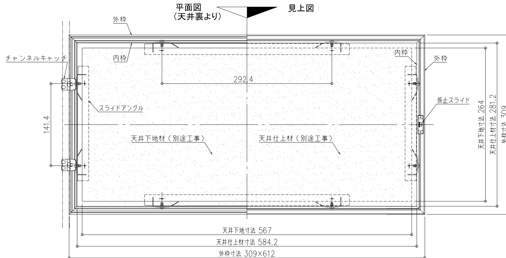
平面・見上図 S=1/4
