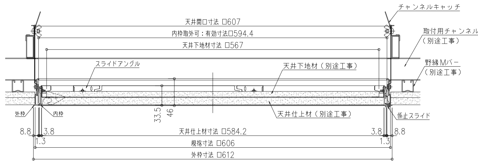
断面図 S=1/4
