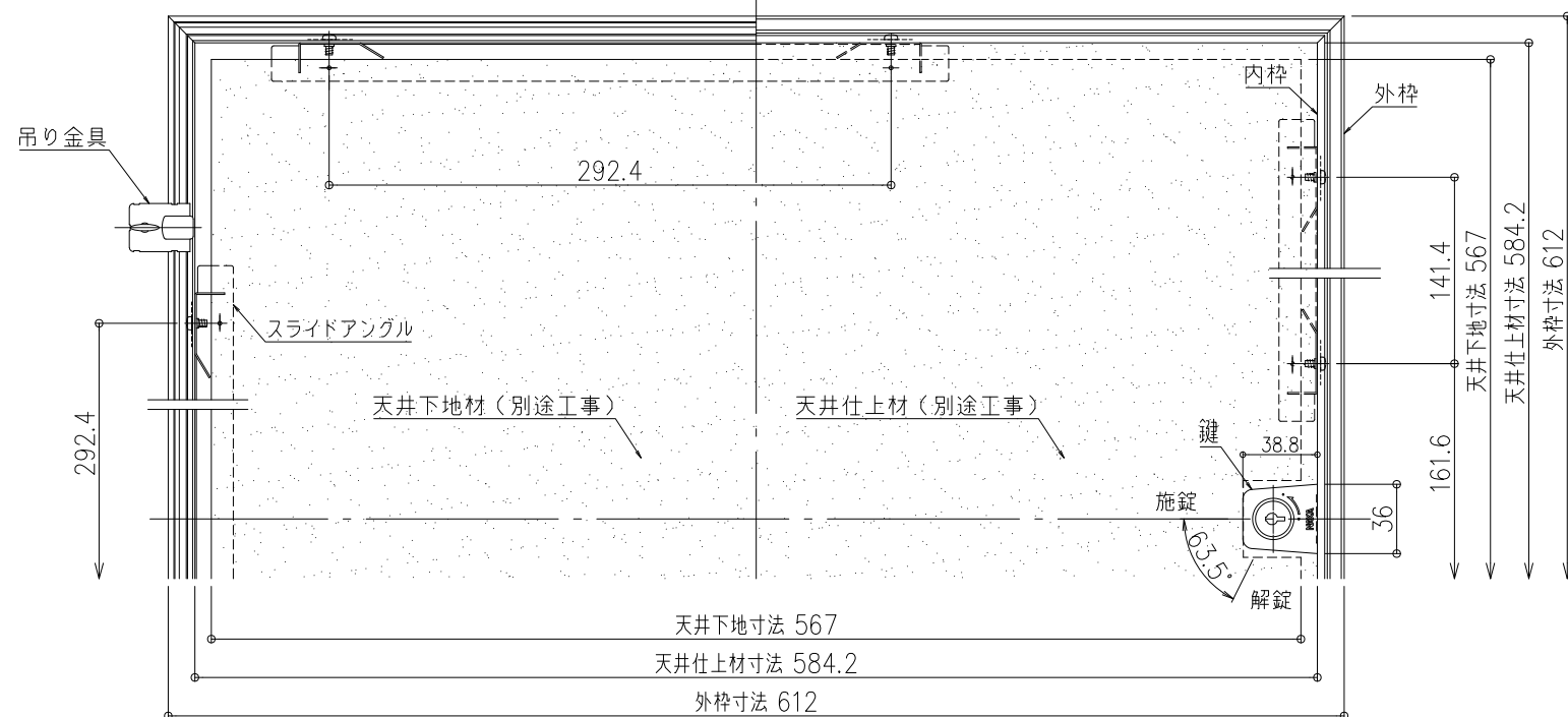
平面・見上図 S=1/4
