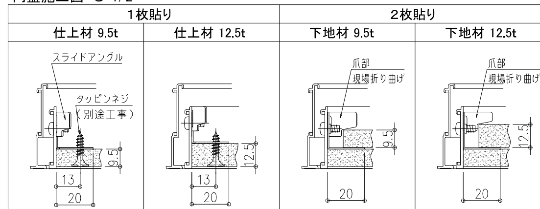
内蓋施工図 S=1/2
