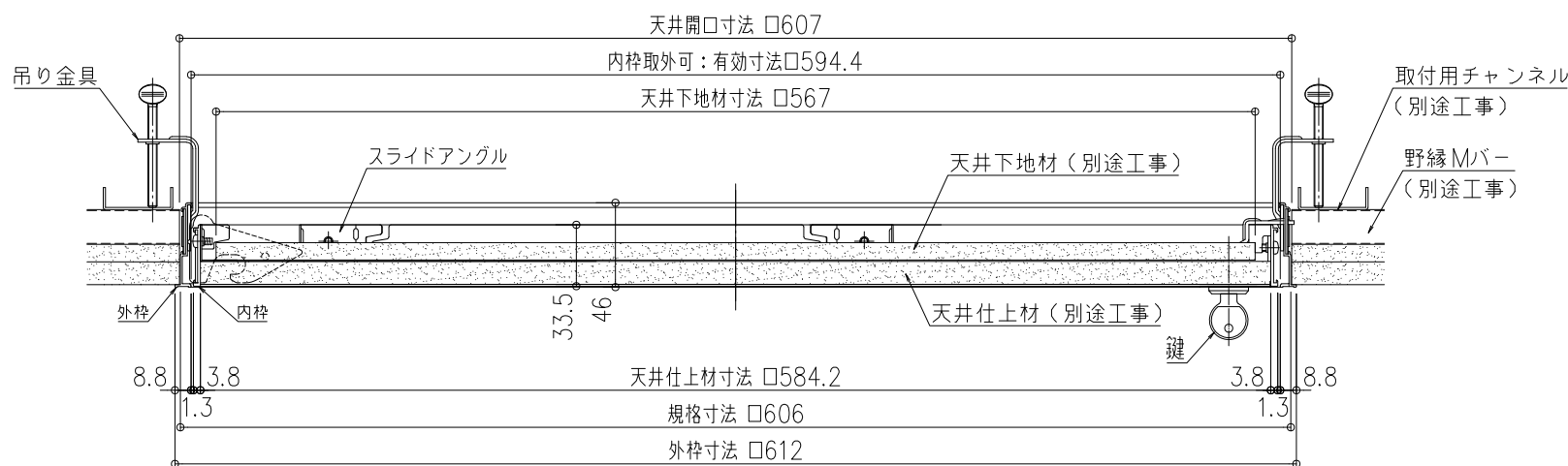
断面図 S=1/4
