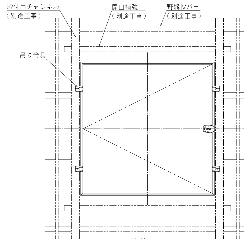
取付状態図 S=1/10
