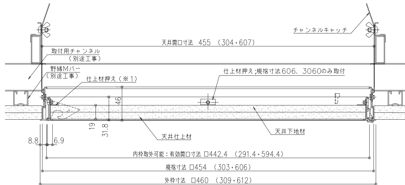
係止部見上げ図 S=1/3
