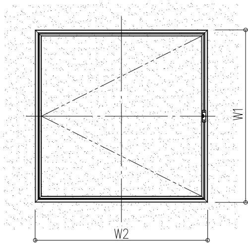
係止スライド仕様伏図 S=1/10
