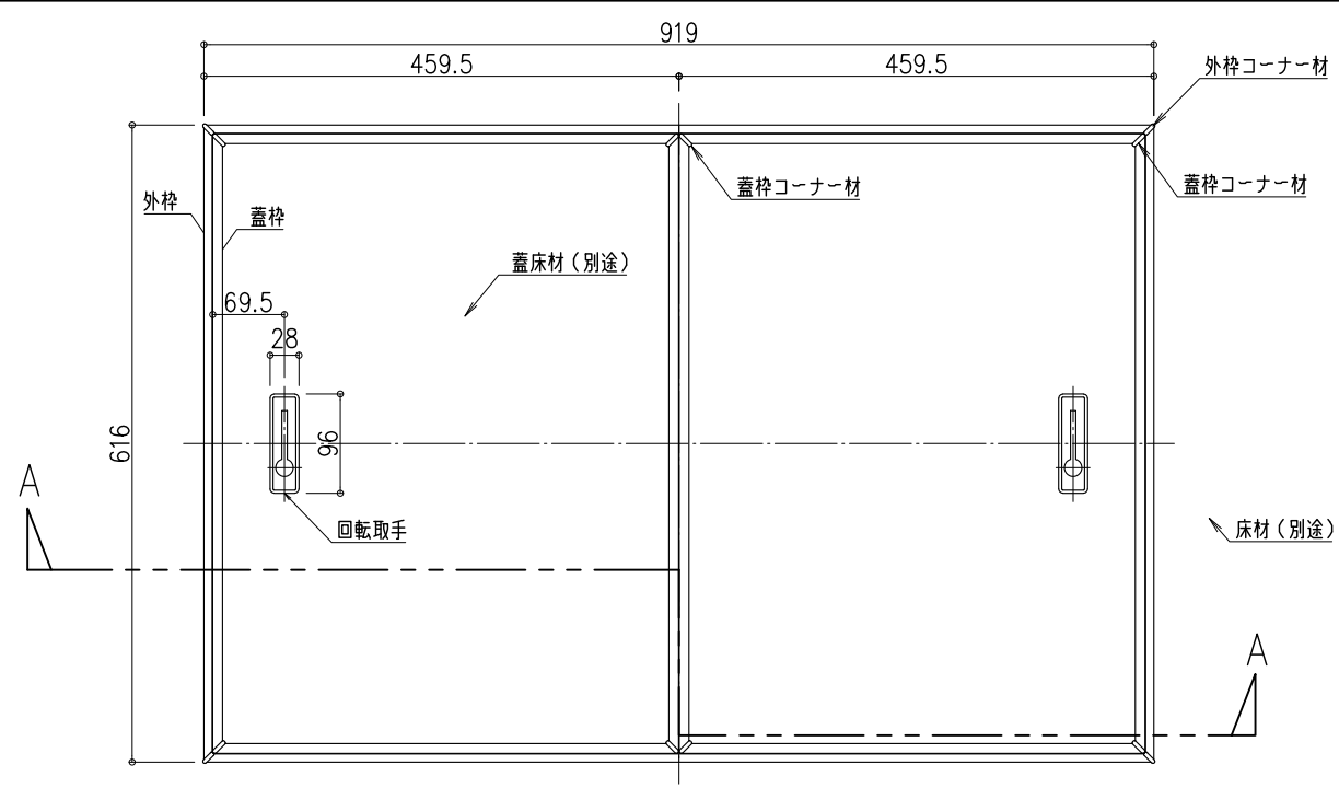
姿図 S=1/8
