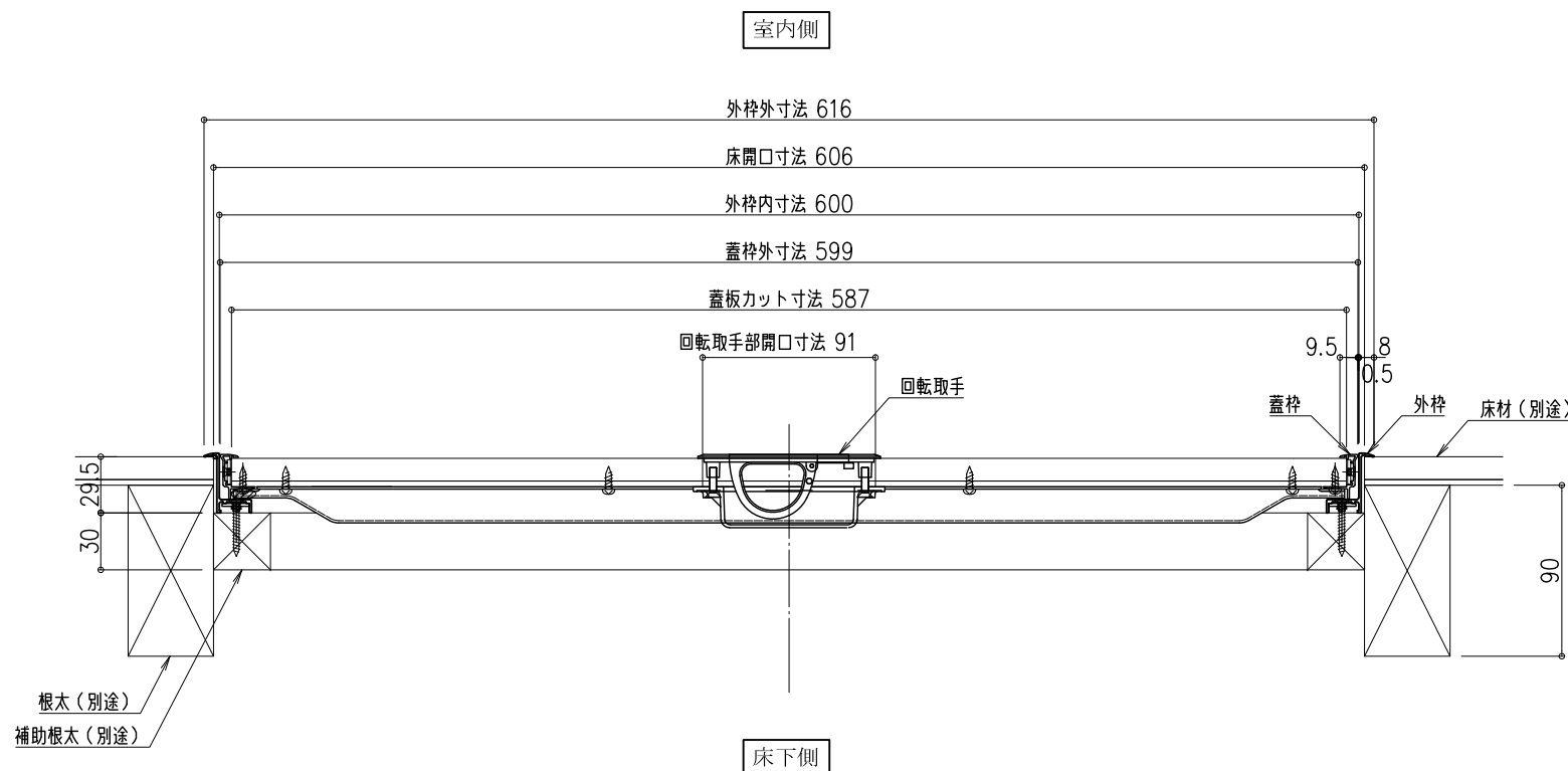
B-B断面詳細図 S=1/4
