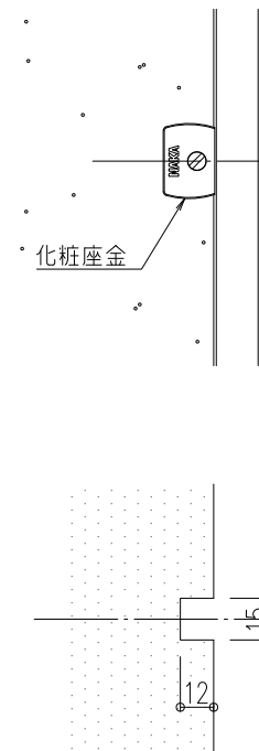
天井仕上材切欠き寸法 (天井下地材の切欠きは不要)
