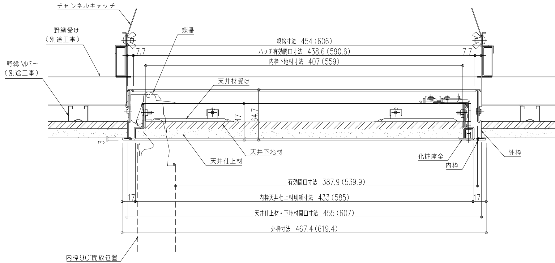
規格寸法・外枠寸法
