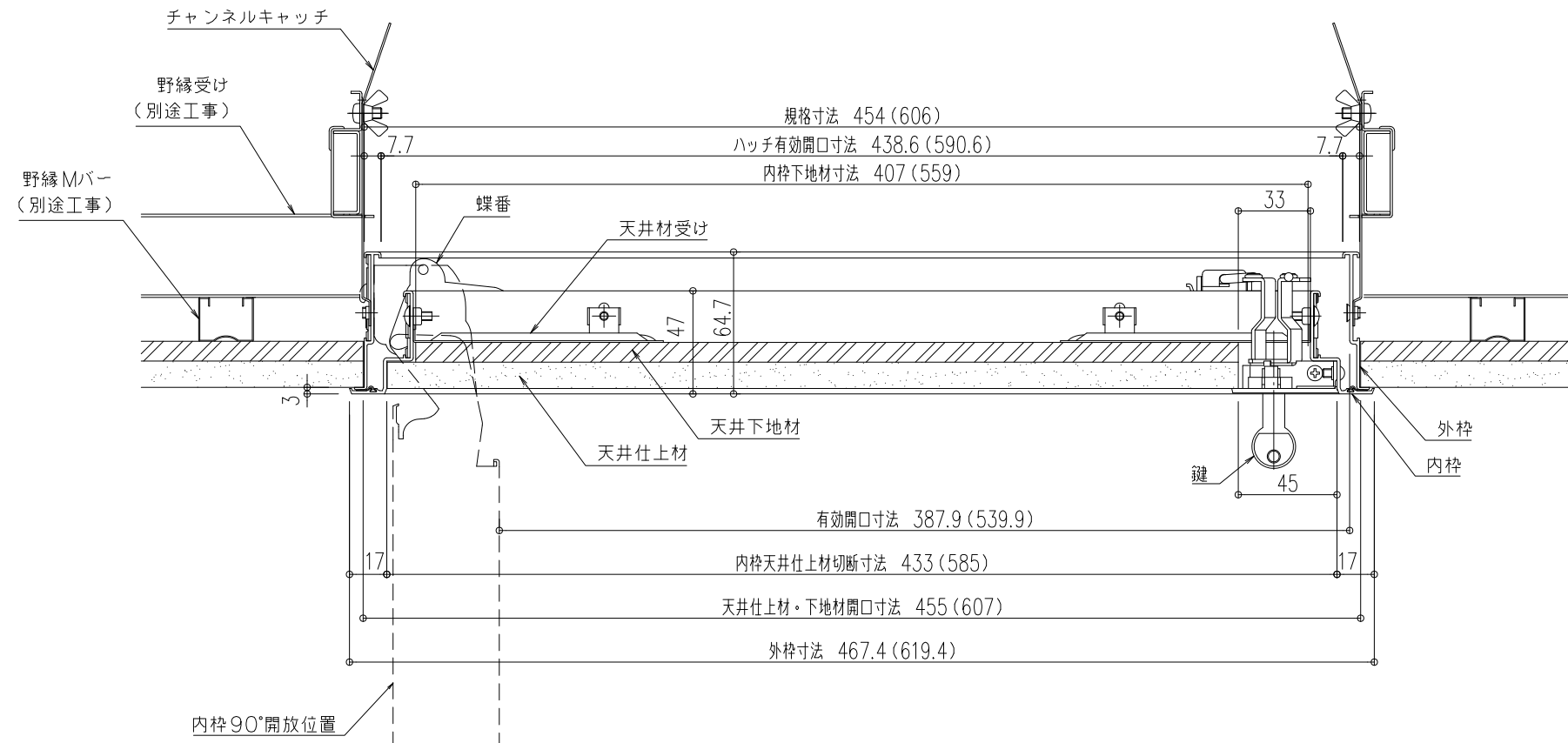
取付下地図 S=1/10 規格寸法・外枠寸法 S=1/10 鍵正面詳細図 S=1/3
