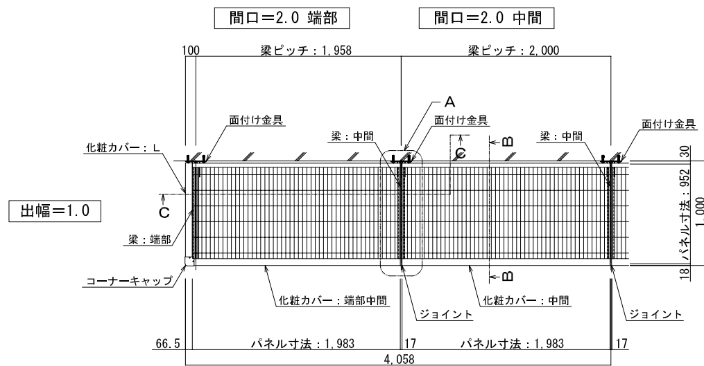
平面図 (1/50)
