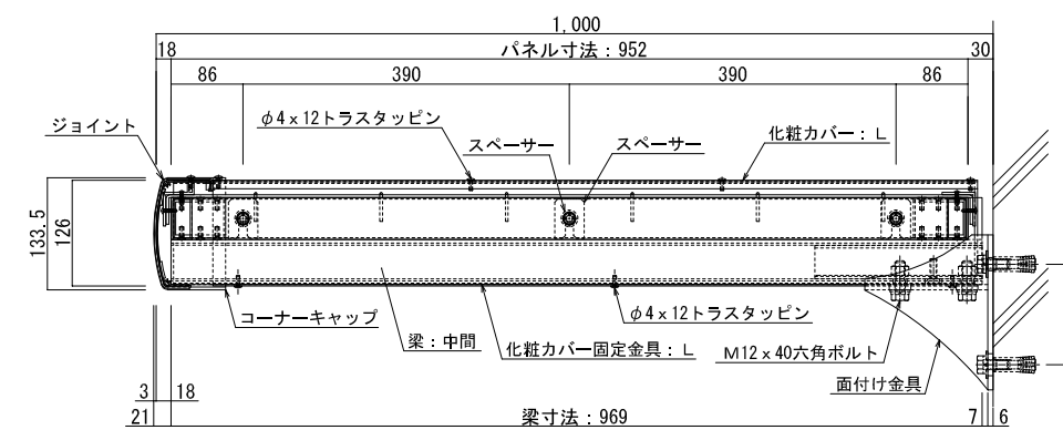
B-B 断面詳細図 (1/10)
