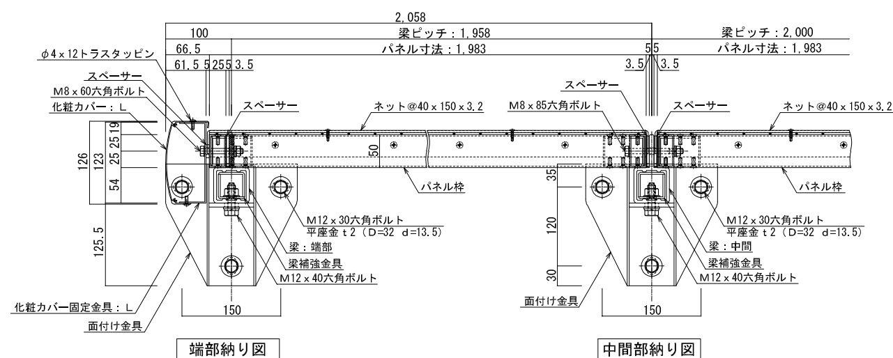
C-C 断面詳細図 (1/8)
