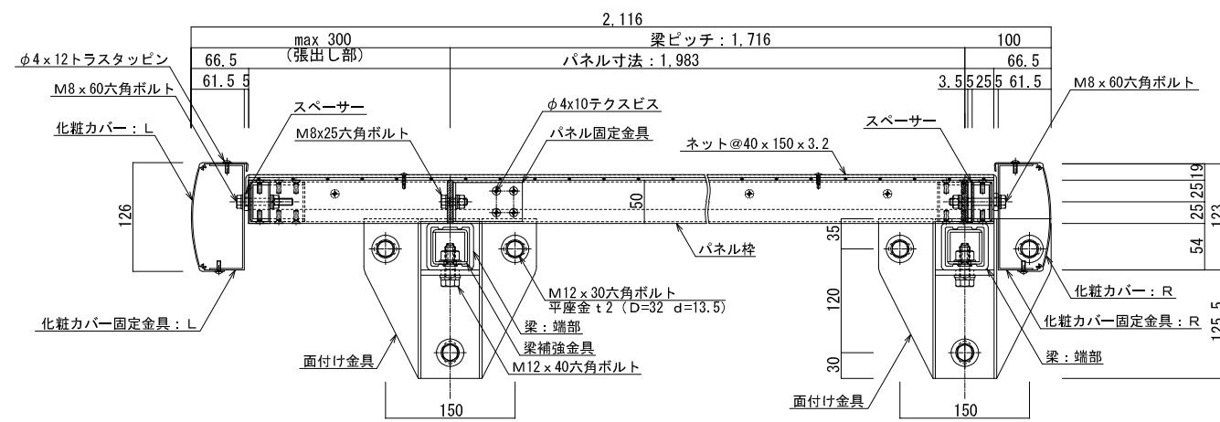
張出し部納り図
