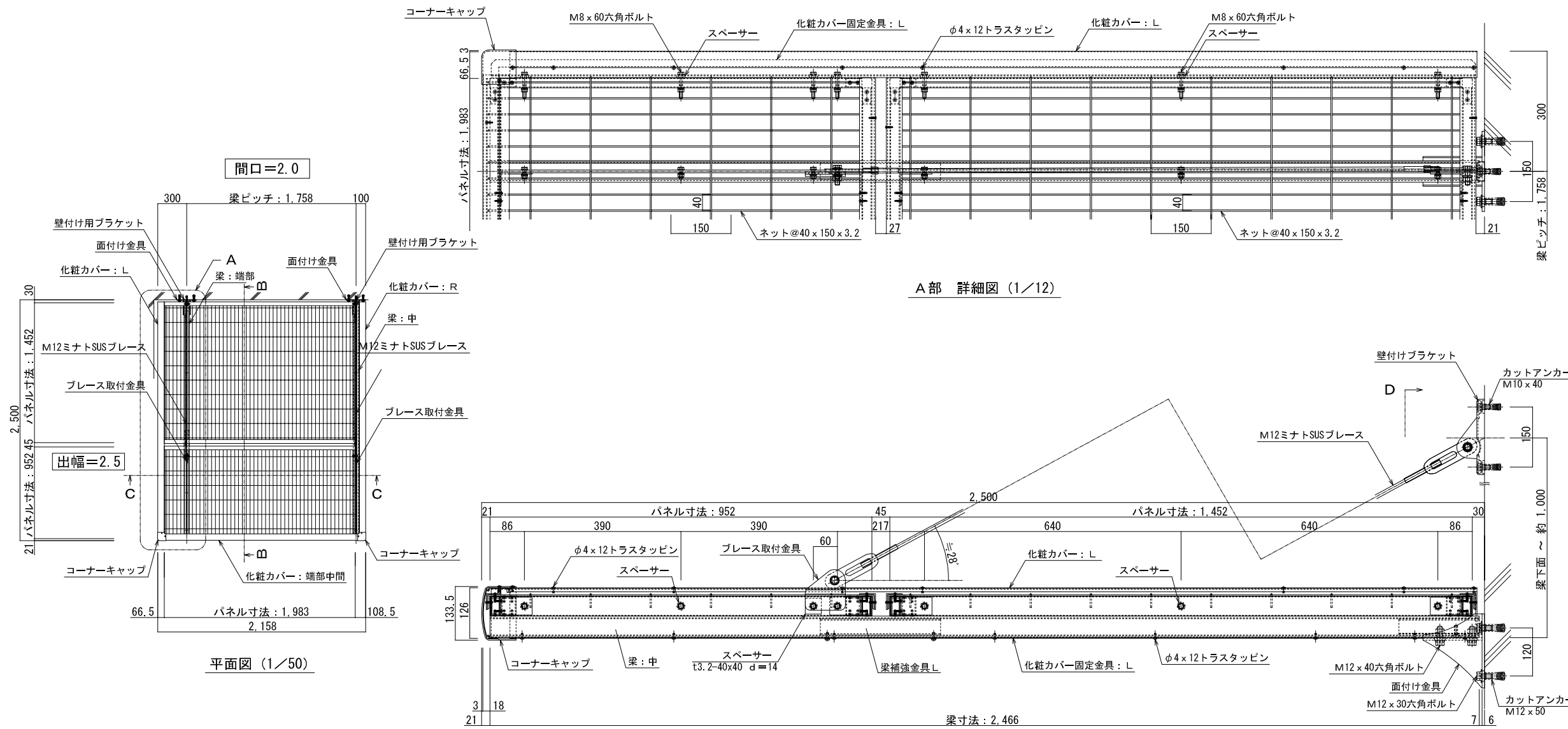
B-B断面詳細図 (1/12)
