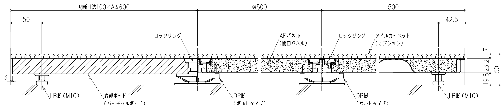
縦断面詳細図 S=1/3
