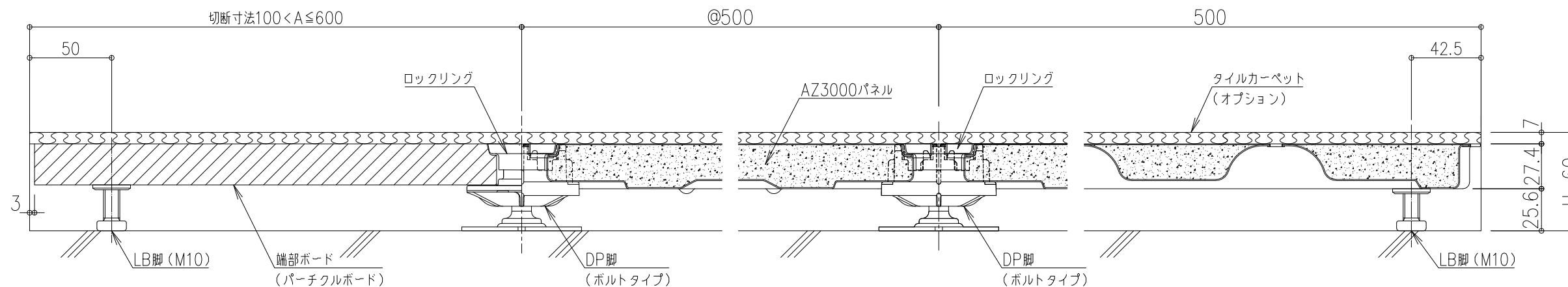
縦断面詳細図 S=1/3
