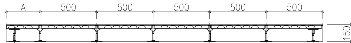
基準納まり図 S=1/20
