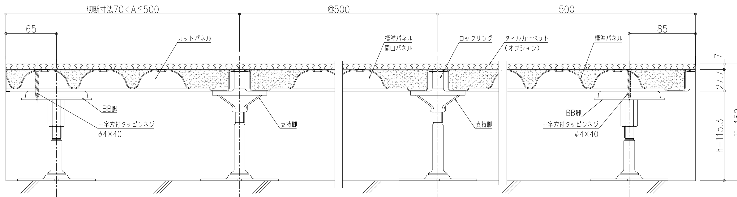
縦断面詳細図 S=1/3
