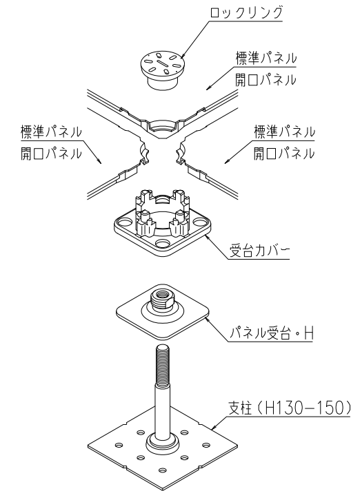
支持脚標準部 納まり図
