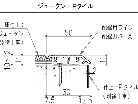
④部 断面図
