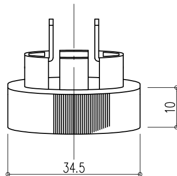
隙間ジョイント外観図 (S=1/1) O-34タイプ 対応用
