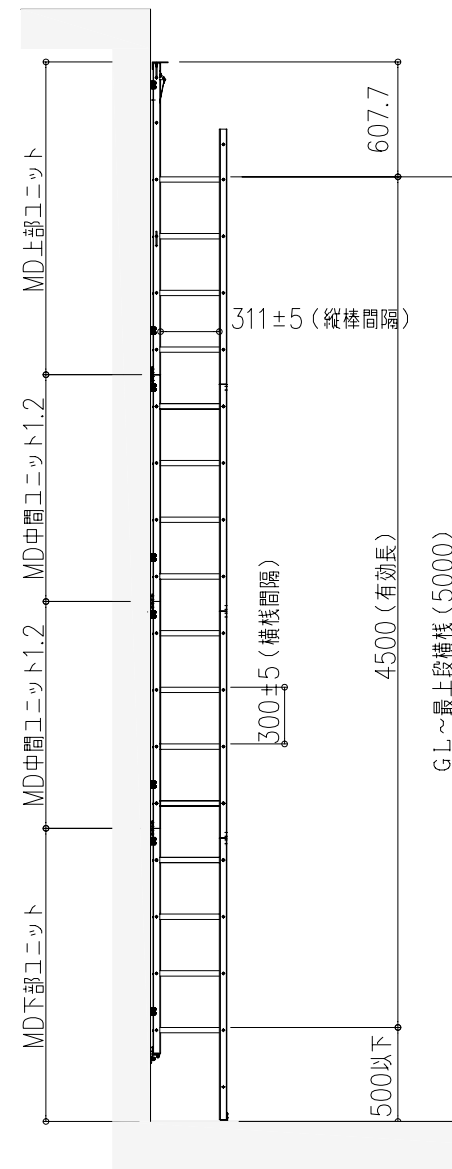
展張時側面
