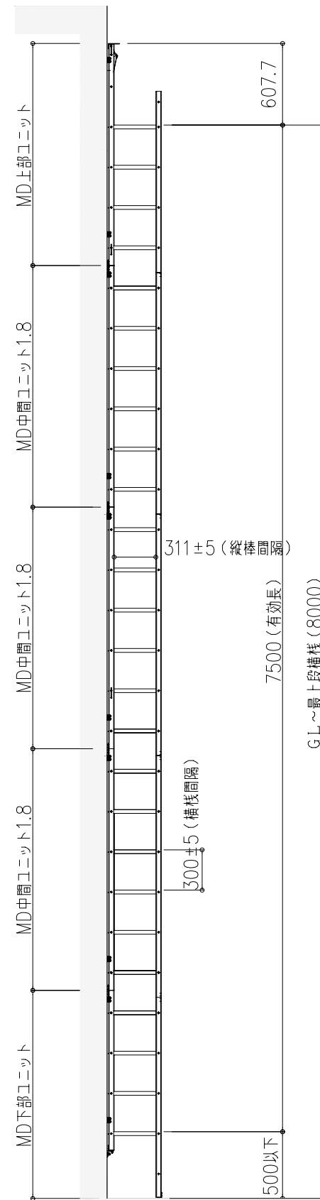
展張時側面
